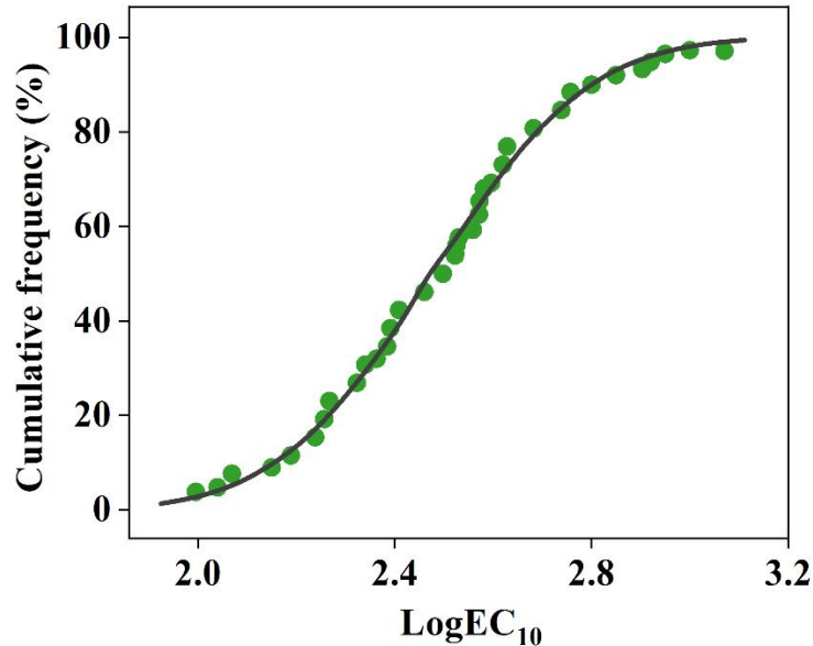
图2 应用物种敏感度分布法推导 HC 5 的示意图
